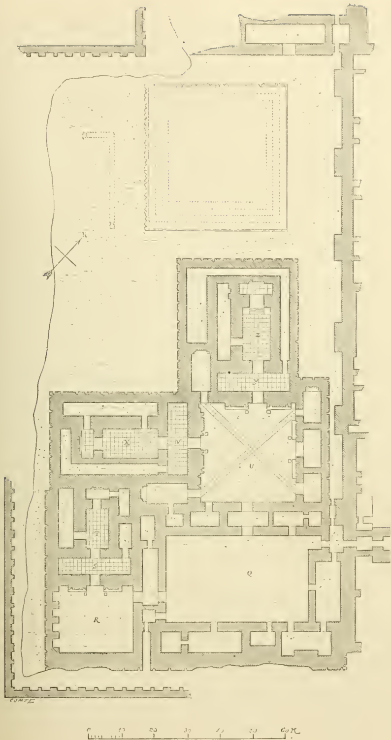
196. — Palais de Sargon. Plan particulier du harem (Place, Niive , t. III, pl. 6).
